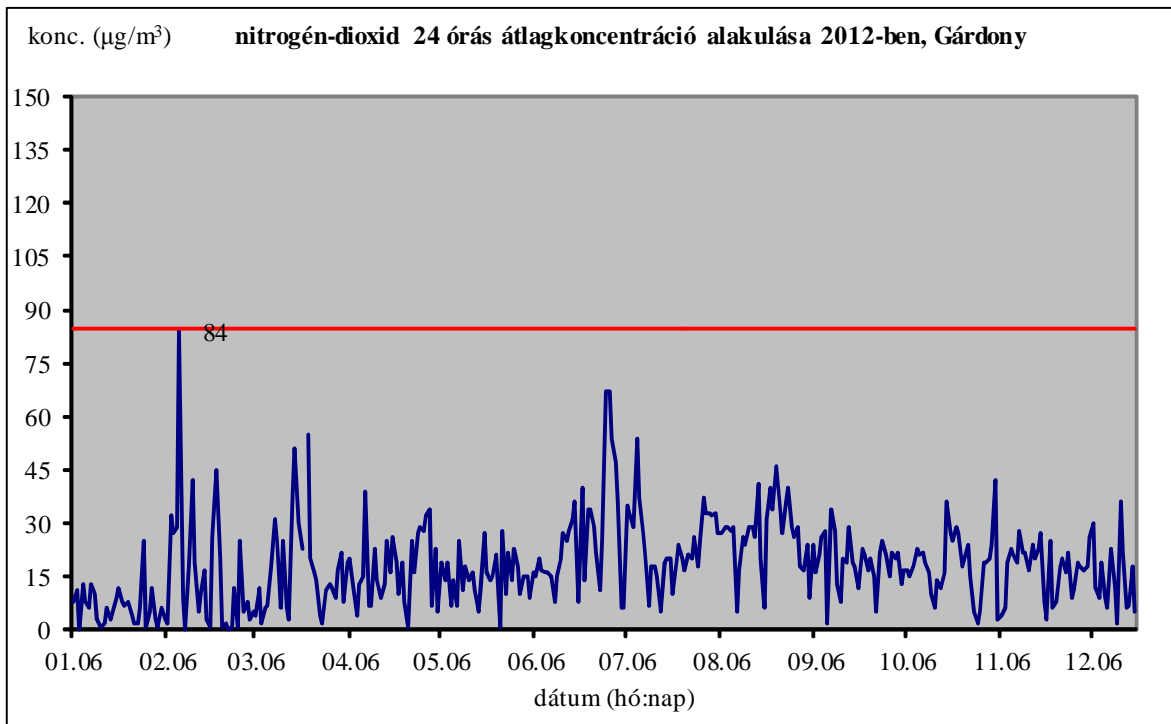
34. ábra. nitrogén-dioxid 24 órás koncentráció átlagának alakulása 2012-ben a Gárdony mérőpon- ton
