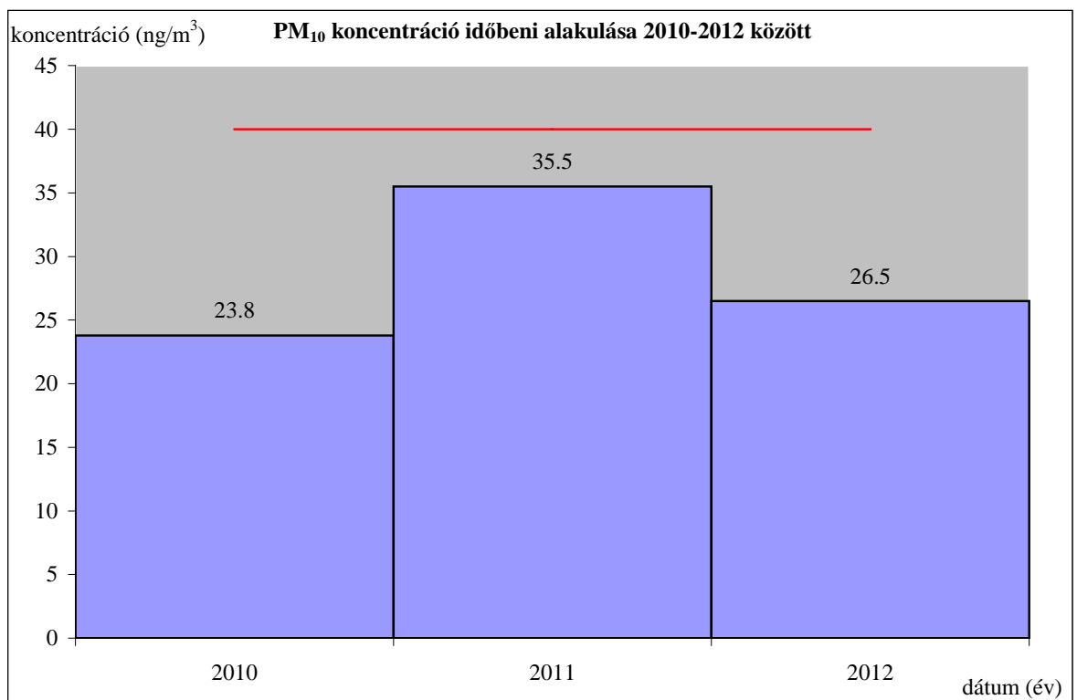
29. ábra: PM 10 éves átlagok az időszakos indikatív mérések eredményei alapján
