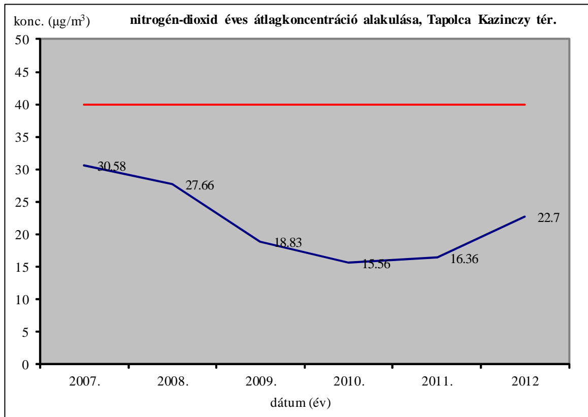
27. ábra. A nitrogén-dioxid éves átlagának menete 2007-2012. között
